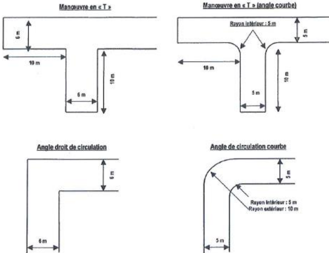
Annexe 4 : schéma des différentes manœuvres des véhicules de collecte
